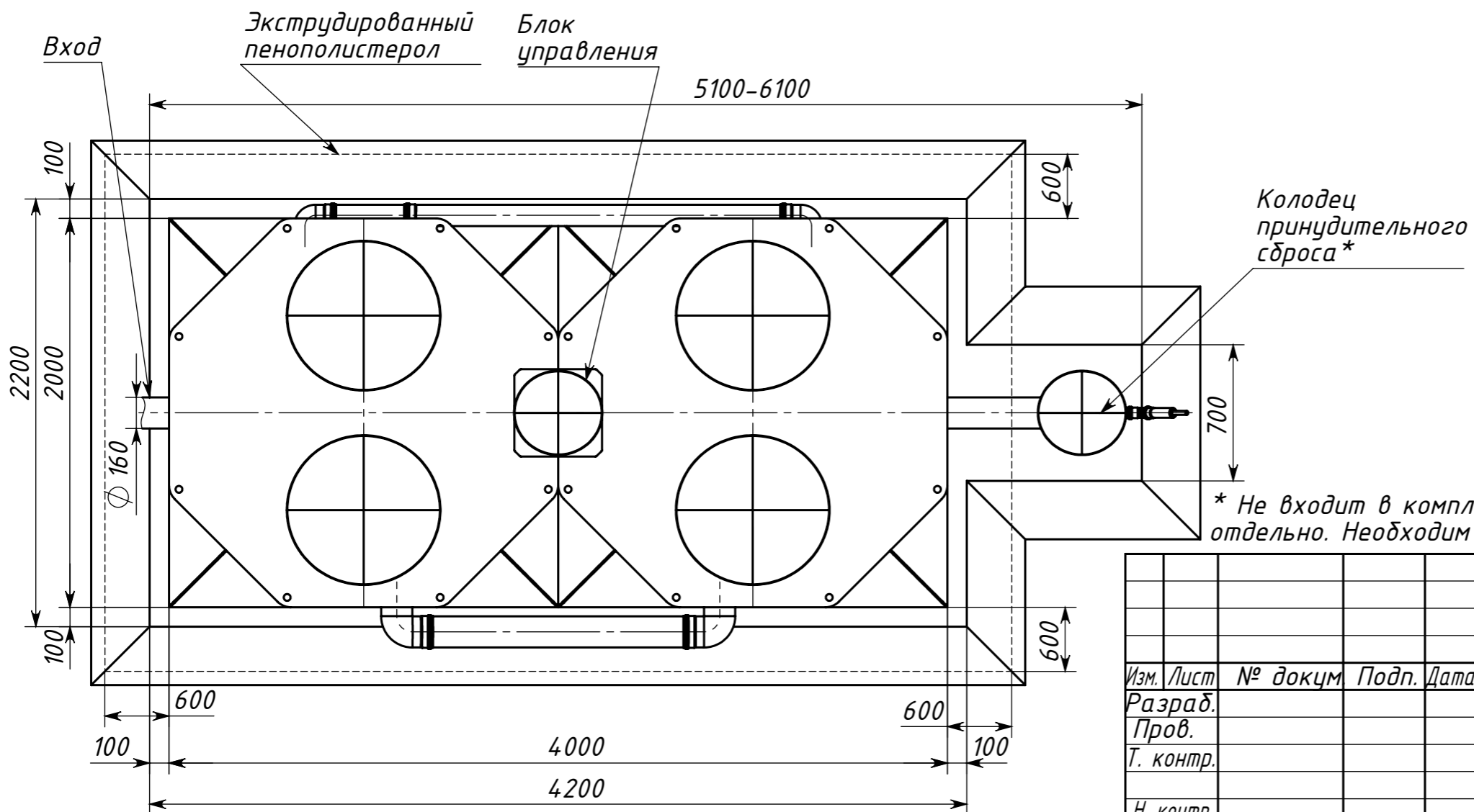
Вид сверху
